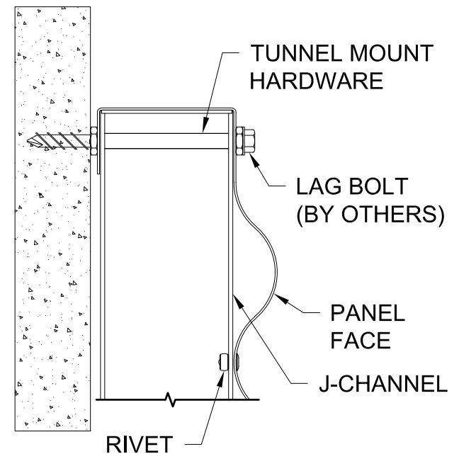
SECTION A-A
